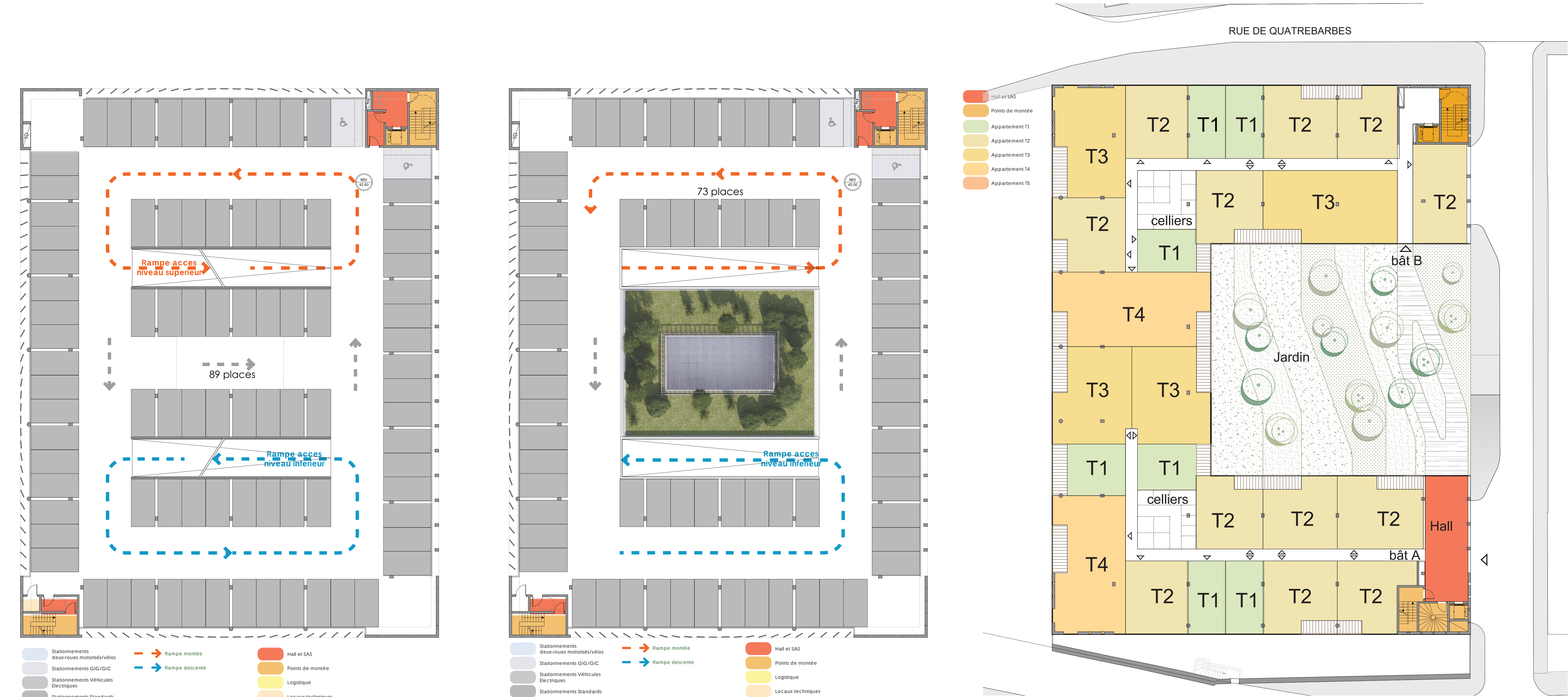
PLAN DE NIVEAU R+1, ECHELLE 1/200ÈME.
