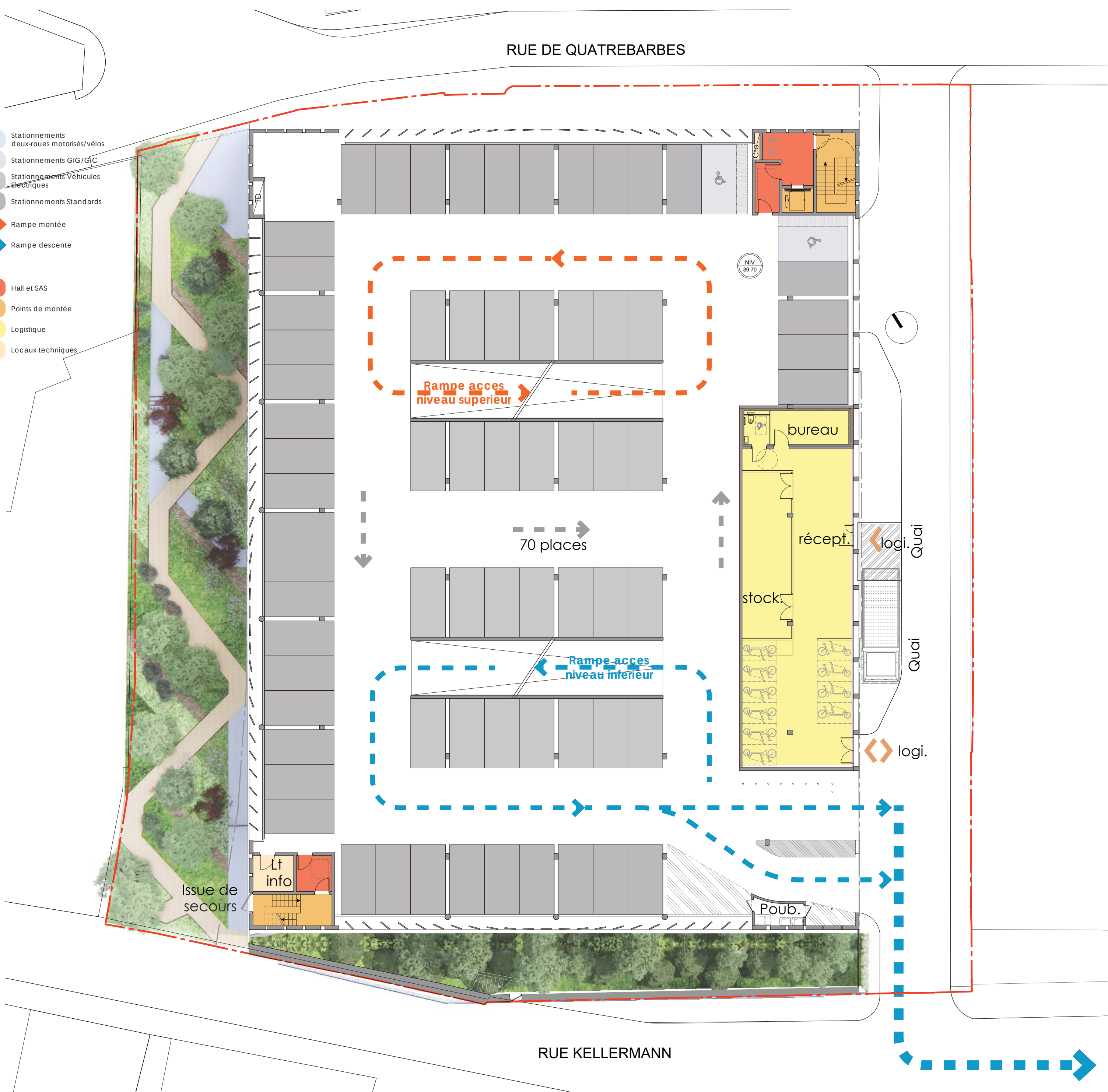
PLAN DE REZ-DE-CHAUSSEE HAUT, ECHELLE 1/200ÈME.
